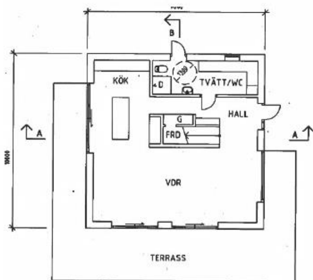
BOTTENVÅNING 1:100
