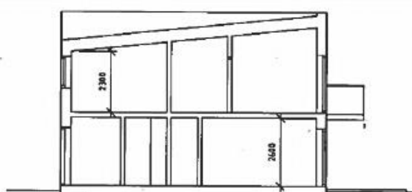
SEKTION B-B 1:100
