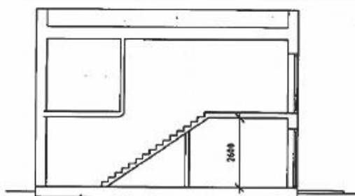
SEKTION A-A 1:100
