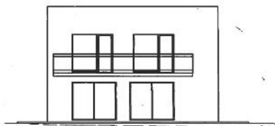
FASAD MOT SÖDER 1:100
