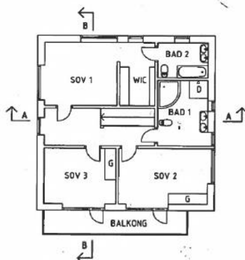
ÖVERVÅNING 1:100
